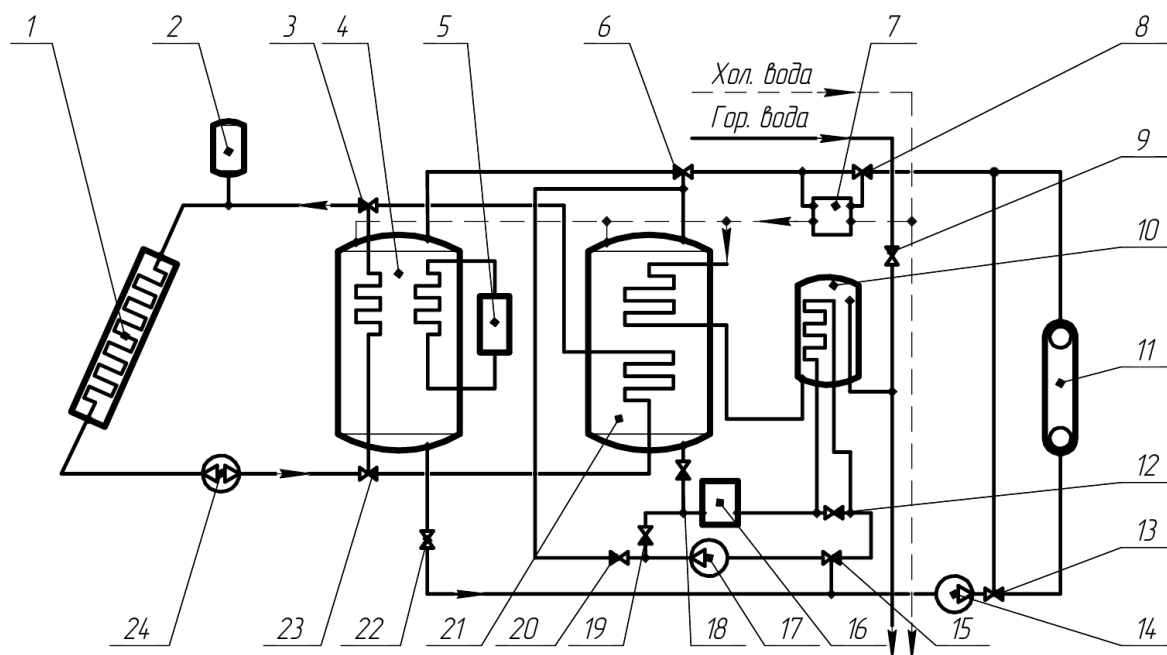
Рис. 1. Двухконтурная ХСИТИ: 1 – радиатор; 2 – расширительный бачок; 3, 6, 8, 13, 15, 23 – гидрораспределители; 4 – аккумулятор холодной воды; 5 – холодильная машина; 7 – система предварительного нагрева водопроводной воды; 9, 12, 18, 19, 20, 22 – вентили; 10 – аккумулятор горячей воды; 11 – система кондиционирования воздуха; 14, 17 – насосы нереверсируемые; 16 – проточный водонагреватель; 21 – аккумулятор теплой воды; 24 – насос реверсируемый
