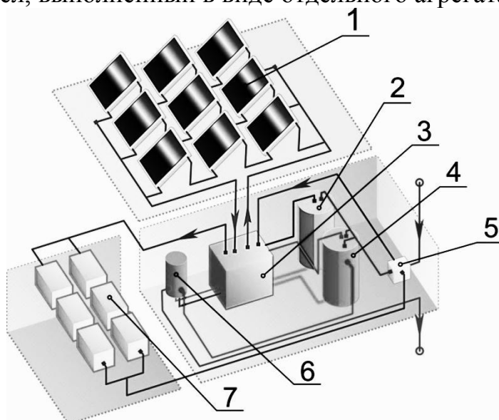
Рис. 2. Система тепло- и хладоснабжения с выделенным агрегатом управления: 1 – радиаторы; 2 – аккумулятор холодной воды; 3 – центральная система управления; 4 – аккумулятор теплой воды; 5 – система предварительного подогрева холодной воды; 6 – аккумулятор горячей воды; 7 – система кондиционирования воздуха.
